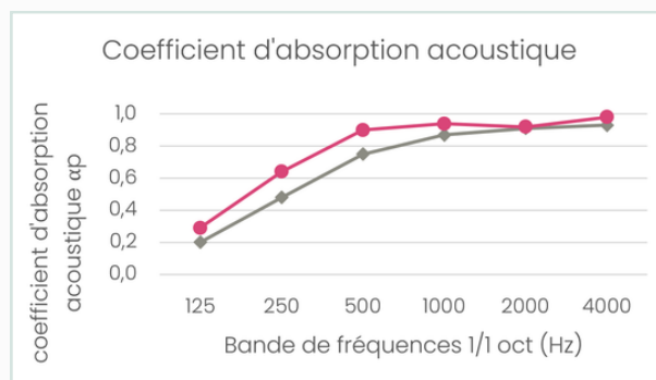
Feutre PET (épaisseur : 40 mm) – montage direct Feutre PET (épaisseur : 40 mm) – lame d'air de 50 mm
