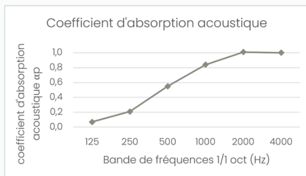
Feutre PET (épaisseur : 25 mm) – montage direct
